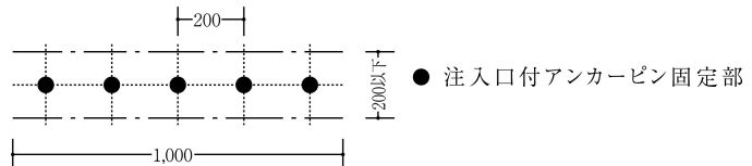
図4.3.3 標準配置グリッド(mm)
