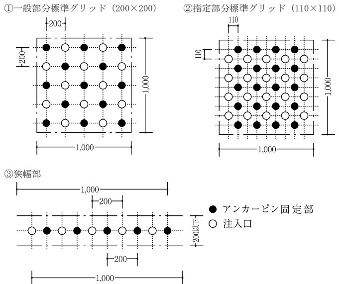
図4.3.2 標準配置グリッド(mm)
