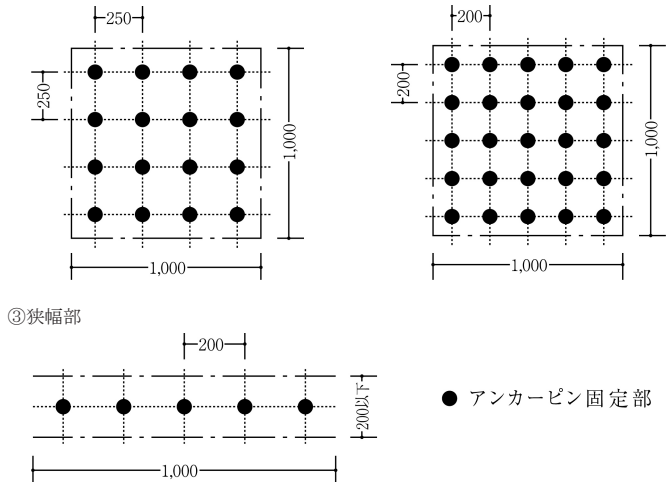
図4.3.1 標準配置グリッド(mm)
