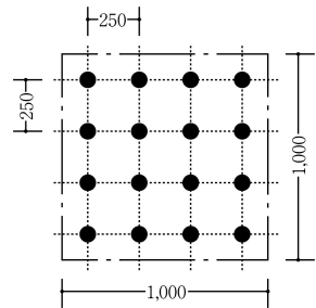
②指定部分標準グリッド (250×250)
